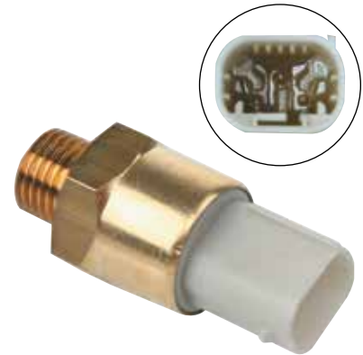
TFS249 Fan Switch
